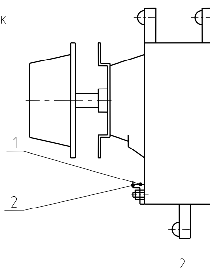
Рис. 4. Термоограничитель АШГ 5.868.000 (только для СЭ – 0,35)
